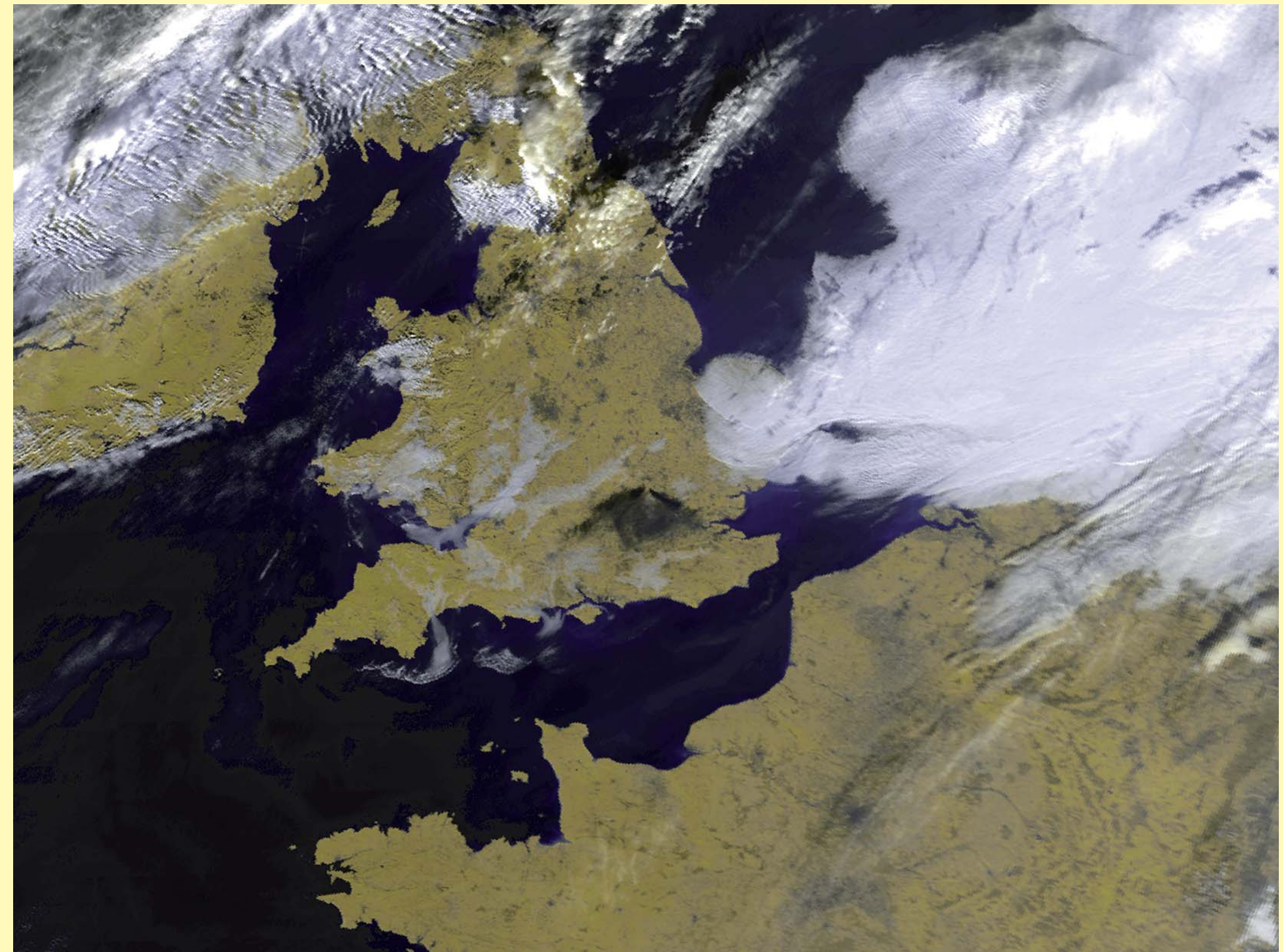
11 décembre 2005 Feux d'hydrocarbures à Londres
