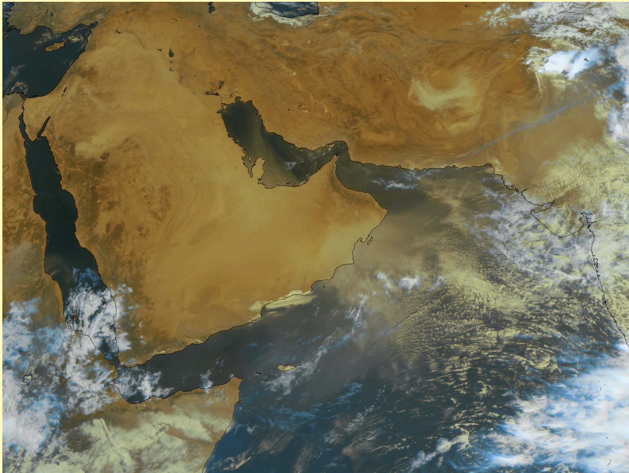
12 juillet 2004 Poussière sur la péninsule arabique
