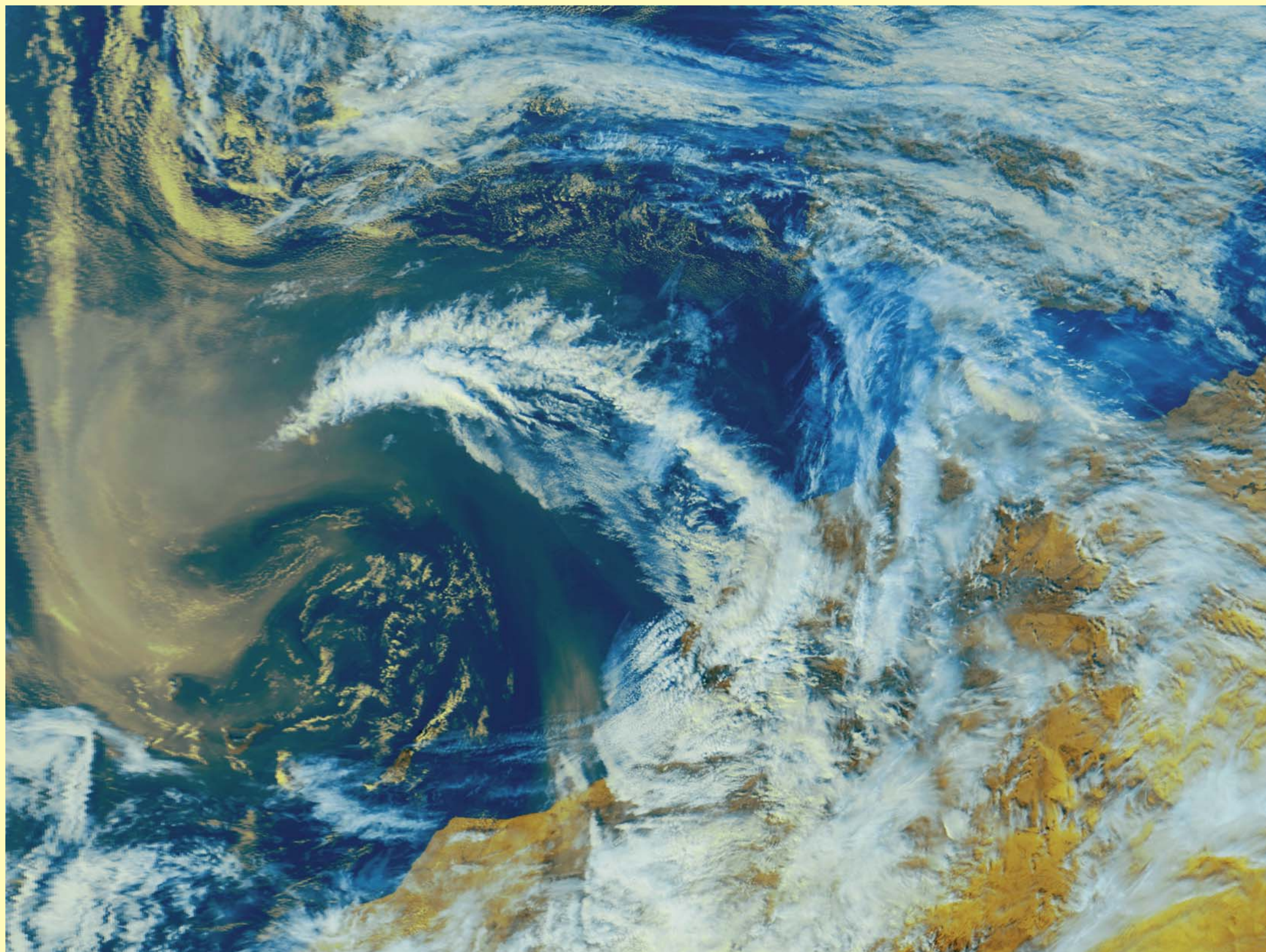
18 février 2004 Transport de poussière sur l'Atlantique
