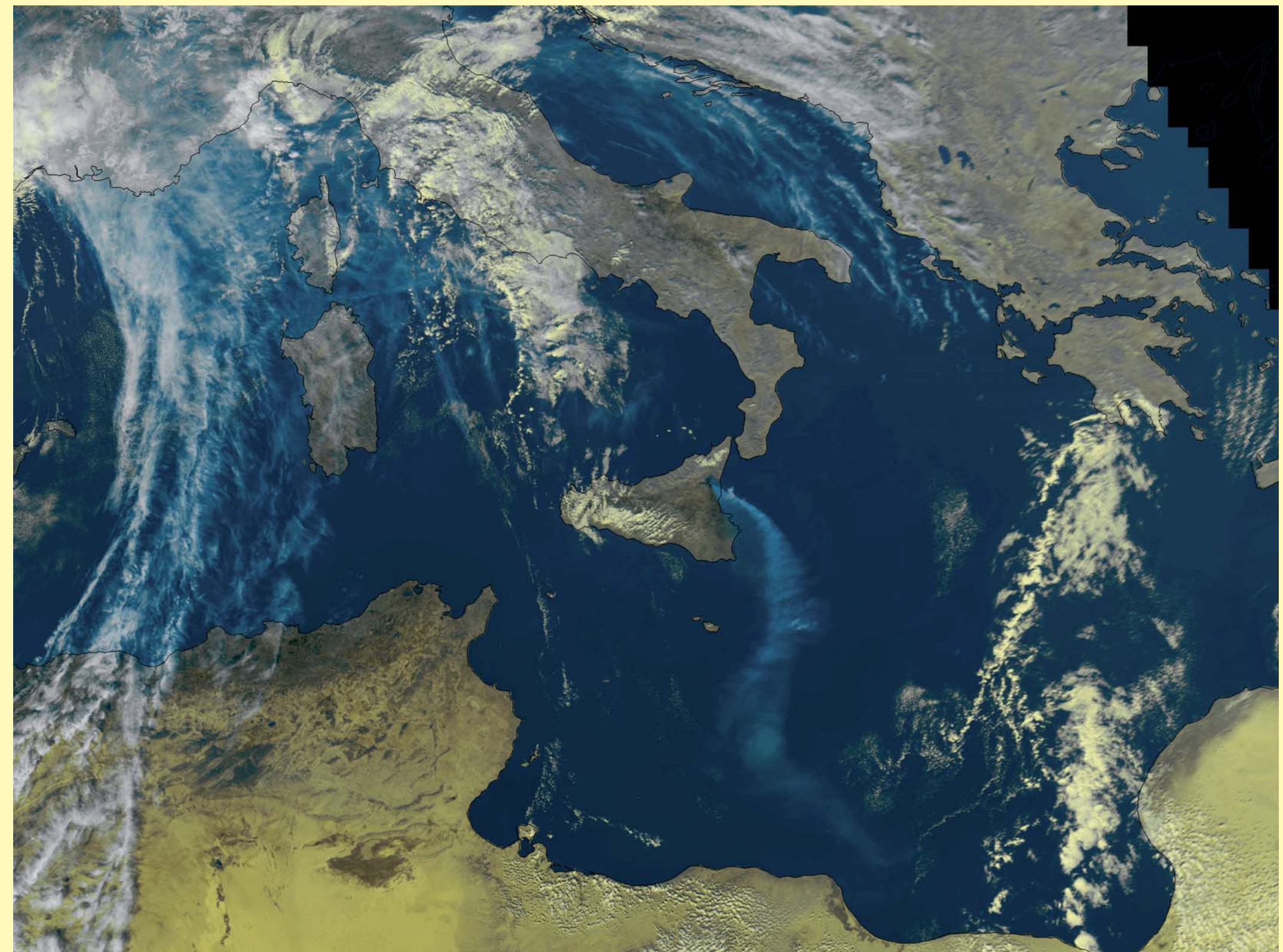
30 octobre 2002 Eruption de l'Etna
