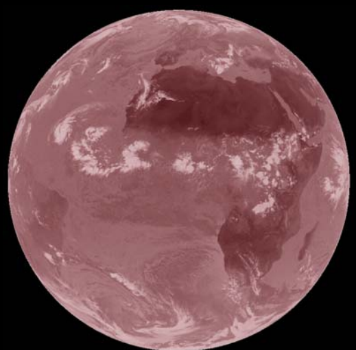
IR 3,9 \mu\text{m}
