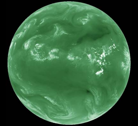
WV 7,3 \mu\text{m}
