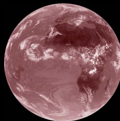
IR 10,8 \mu\text{m}
