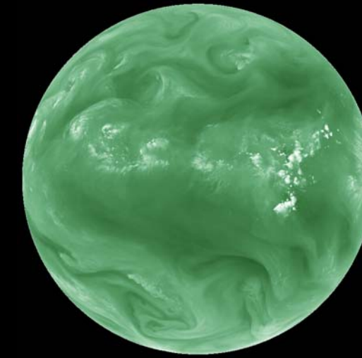
WV 6,2 \mu\text{m}
