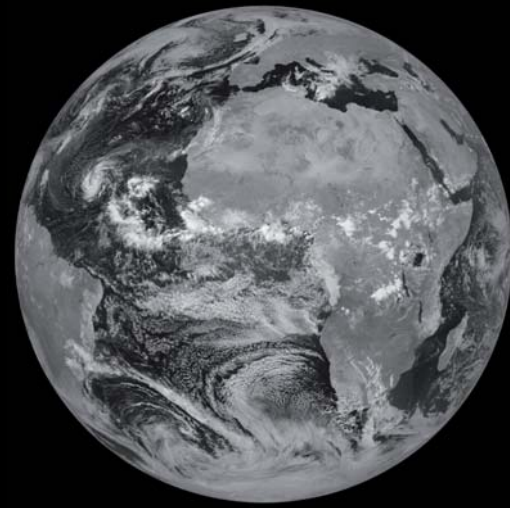
VIS 0,8 \mu\text{m}
