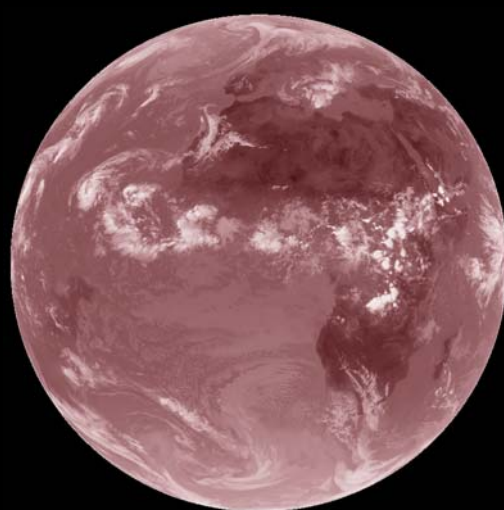
IR 8,7 \mu\text{m}
