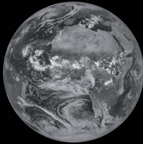
VIS 0,6 \mu\text{m}
