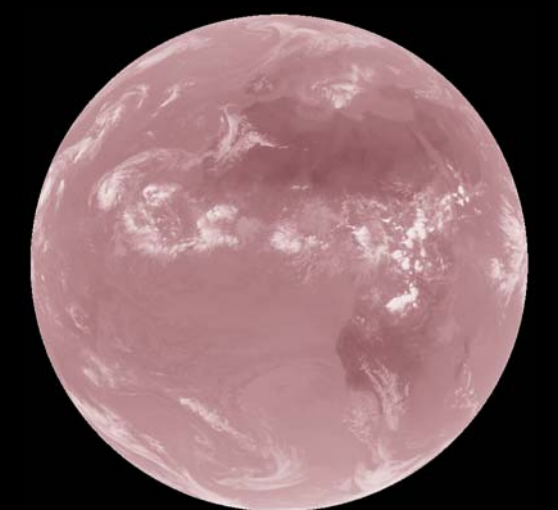
IR 13,4 \mu\text{m}
