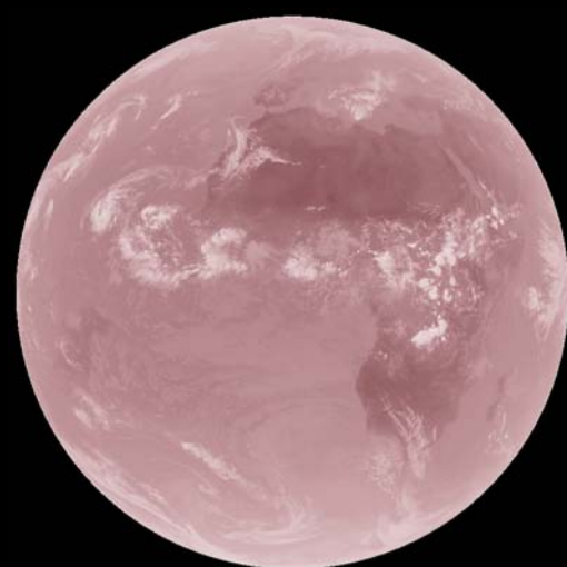
IR 9,7 \mu\text{m}
