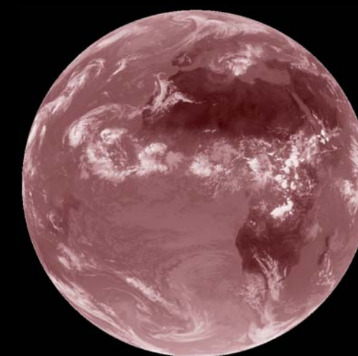
IR 12,0 \mu\text{m}
