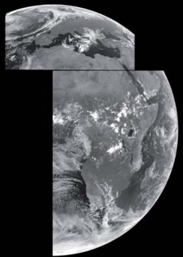
HRV
