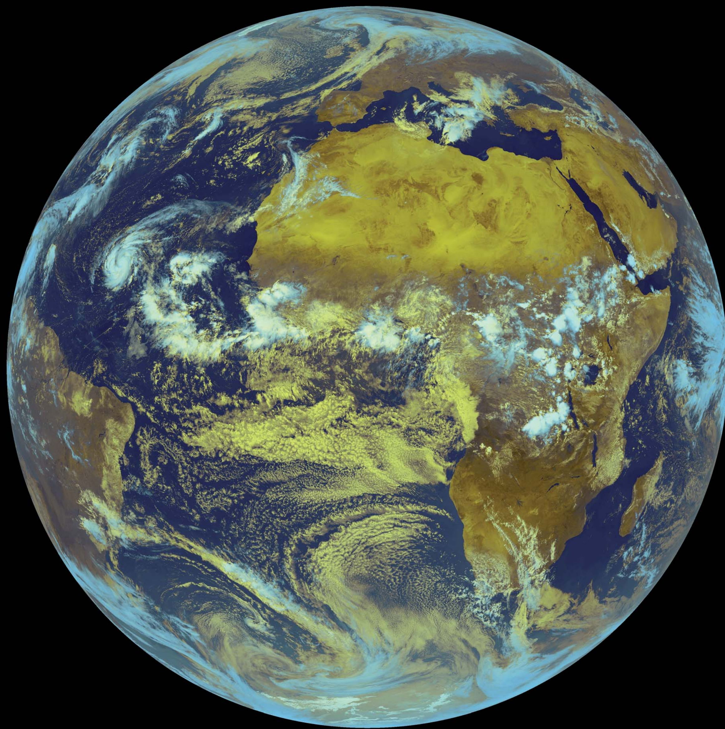
VIS 0,6 \mu\text{m}
